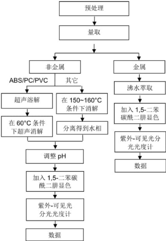
六价铬检测流程图
