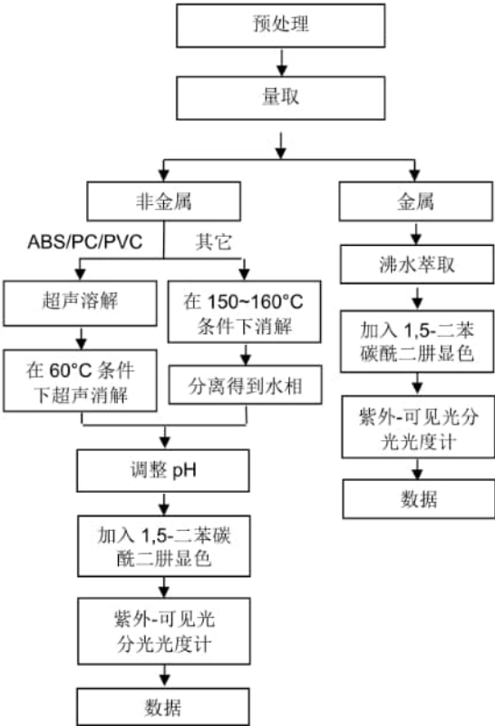
六价铬检测流程图
