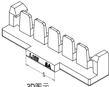
3D图示
