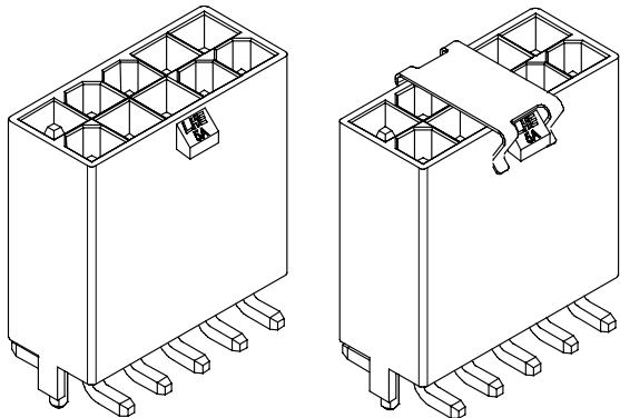
3D图示
