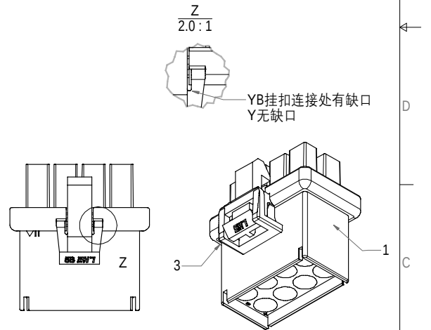
3D图示
