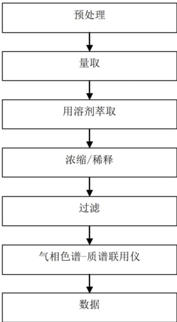
Phthalates 测试流程图
