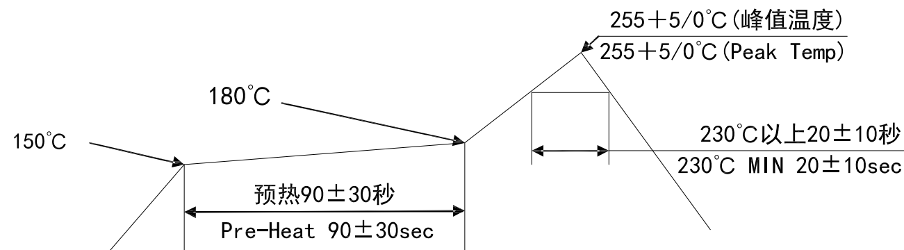
温度条件图
